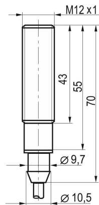
Габаритный чертеж
